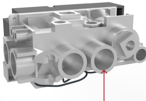
Ø12 mm 3/8" gasinlaat - Alleen als de flexibele leiding niet wordt gebruikt.
