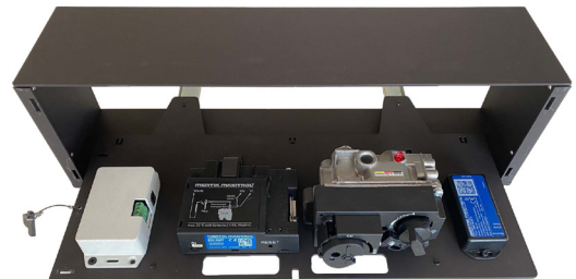
Groot inspectierooster - binnenin
