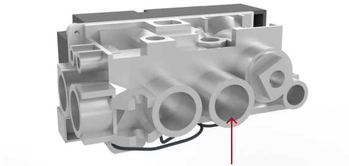
Ø12 mm 3/8" gasinlaat - Alleen als de flexibele leiding niet wordt gebruikt.
